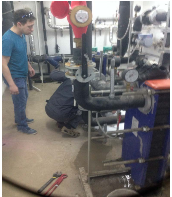
Промывка ИТП.
